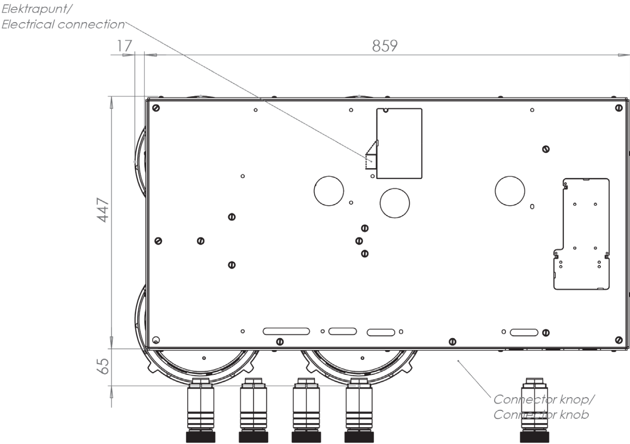
Onderaanzicht / Bottom view
