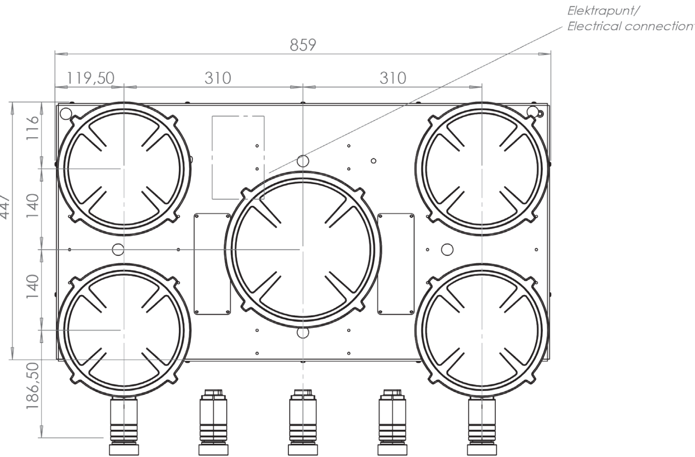
Bovenaanzicht / Top view
