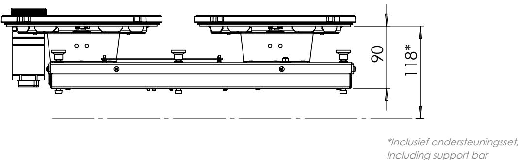
Zijaanzicht / Side view
