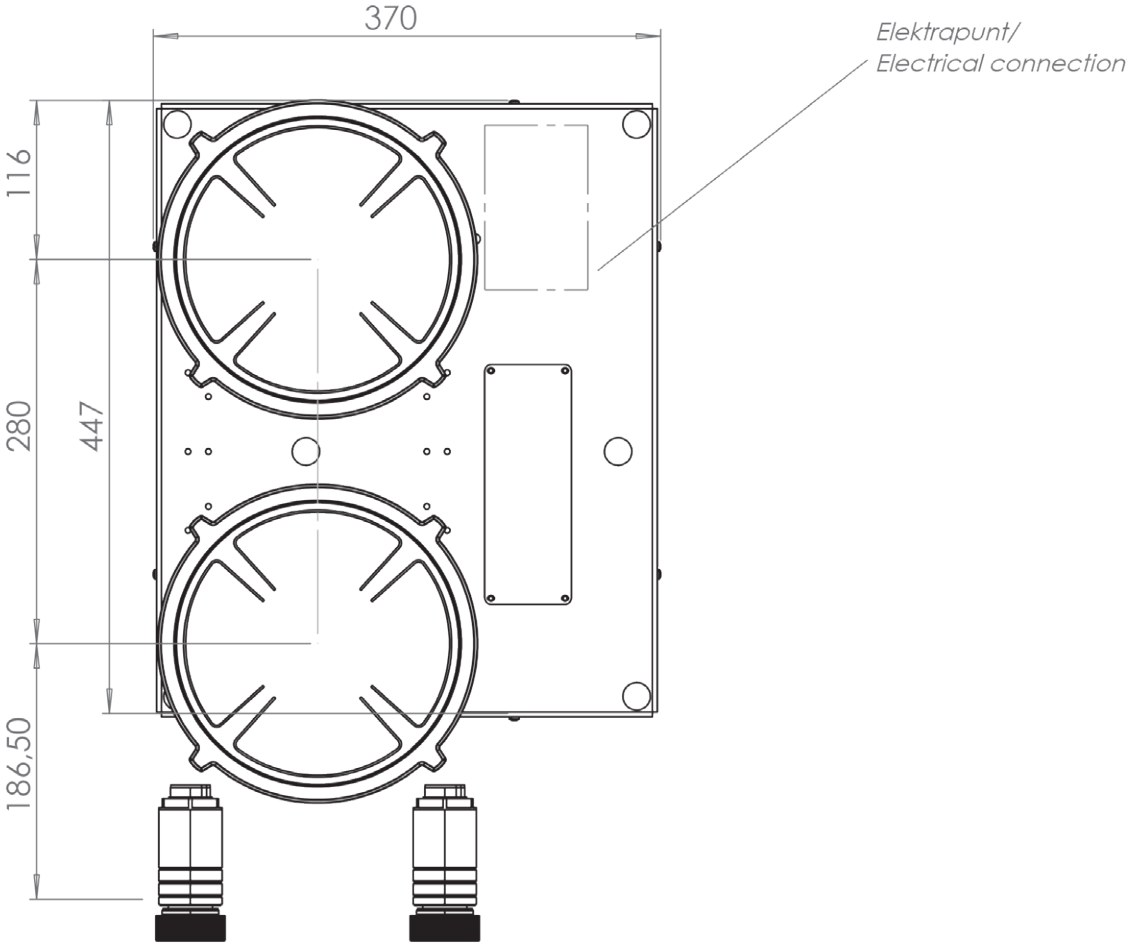
Bovenaanzicht / Top view
